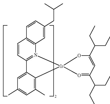
Compound E11
