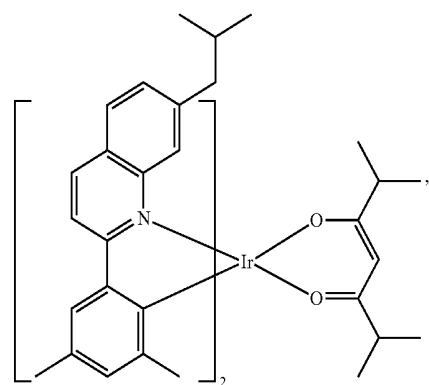
Compound E12
