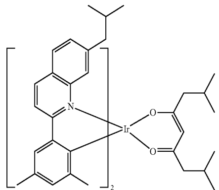
Compound E13
